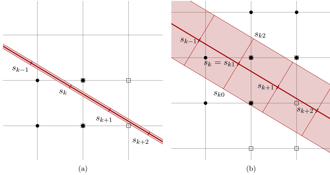
FIGURE 6.7 – Discrétisation du terme d'attache aux microtubules. \bullet : points de grille utilisés pour calculer la valeur de m^* en s_k . \square : en s_{k+1} . 6.7(a) : cas rencontré dans les simulations, où la dimension de la zone d'attraction des microtubules est petite devant le maillage. Seule la valeur en s_k est utilisée pour calculer l'intégrale sur D(s_k) . 6.7(b) : cas où cette dimension a été exagérée et la formule d'intégration implique trois points.
