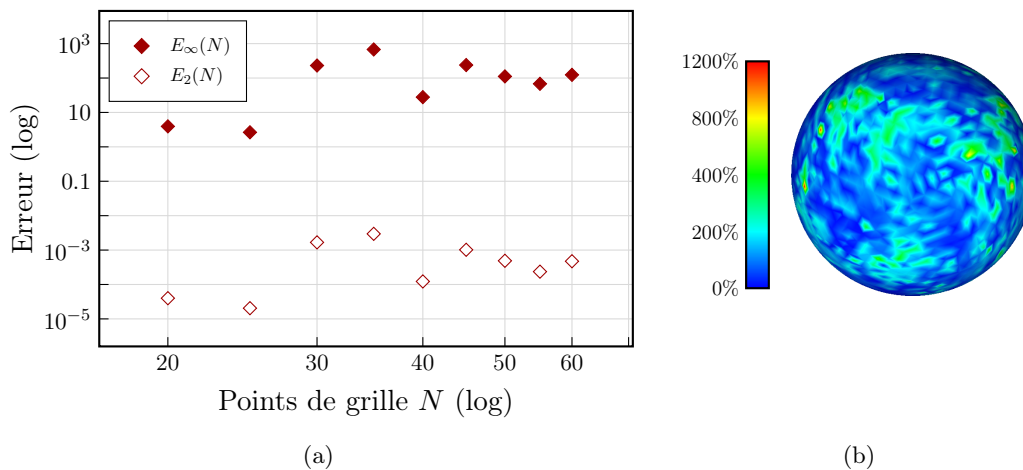
FIGURE 7.2 – 7.2(a) : Non convergence de la discrétisation de l'opérateur de Laplace-Beltrami sur la sphère par la méthode de volumes finis proposée par Xu [99], appliquée au maillage issu de l'intersection de la grille cartésienne et du niveau 0 de la level-set. L'erreur est définie en équation (7.5). 7.2(b) : répartition spatiale de la quantité |\psi - \Psi|_2 / |\mathbf{M}|_2 sur la sphère pour N = 50 .
