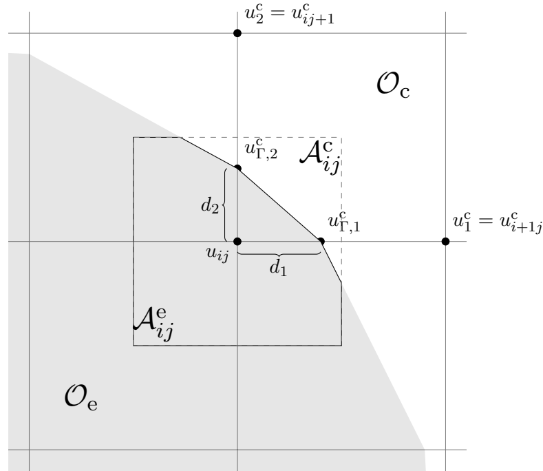
FIGURE 8.4 – Calcul de la norme L^2 sur les points de grille. La valeur de u_{ij}^c est extrapolée à partir de u_1^c , u_{\Gamma,1}^c , u_{\Gamma,2}^c et u_2^c .
