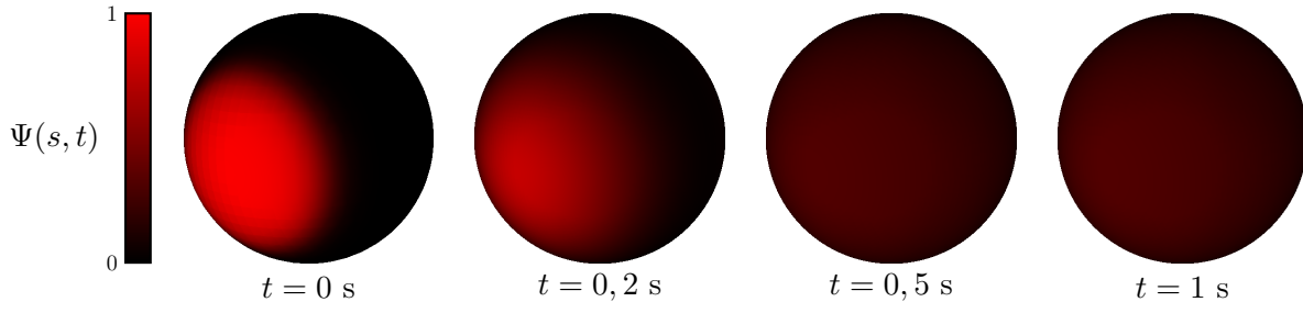
FIGURE 7.10 – Diffusion sur la sphère de la quantité f_2 définie à l'équation (7.9), calculée avec la méthode de différences finies.
